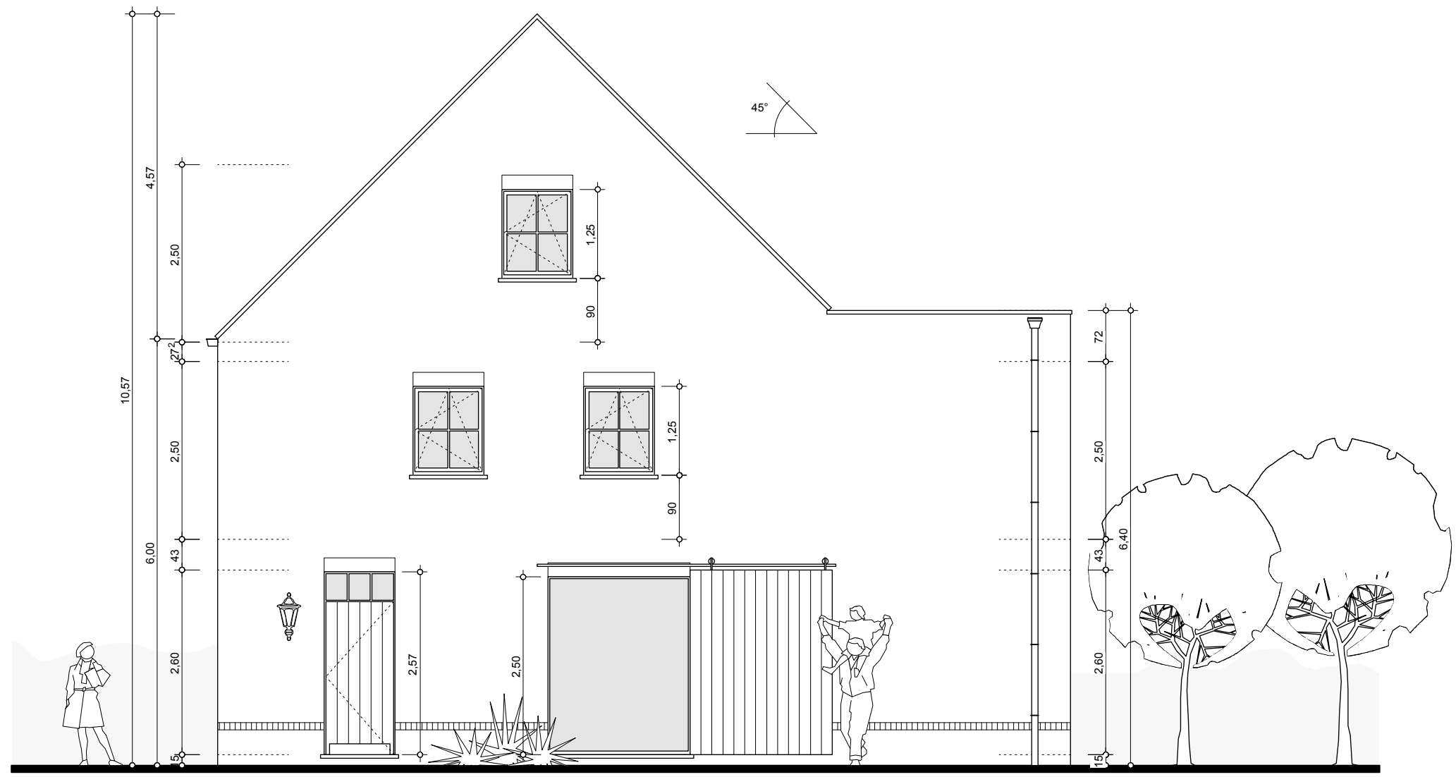
ZIJGEVEL RECHTS schaal: 1/75
